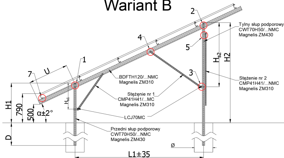
Рис. 1. Боковий вигляд конструкції
