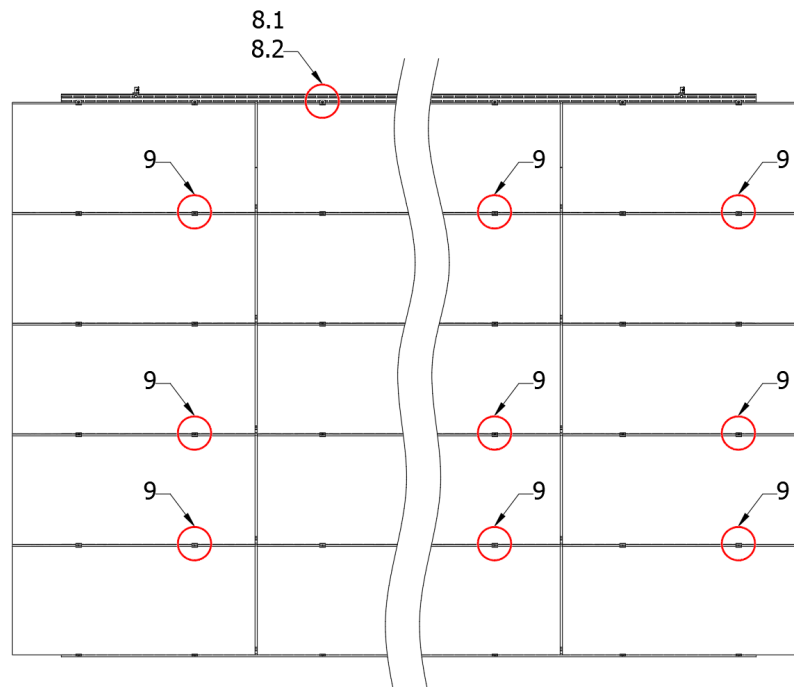
Рис. 4. Вид конструкції зверху
