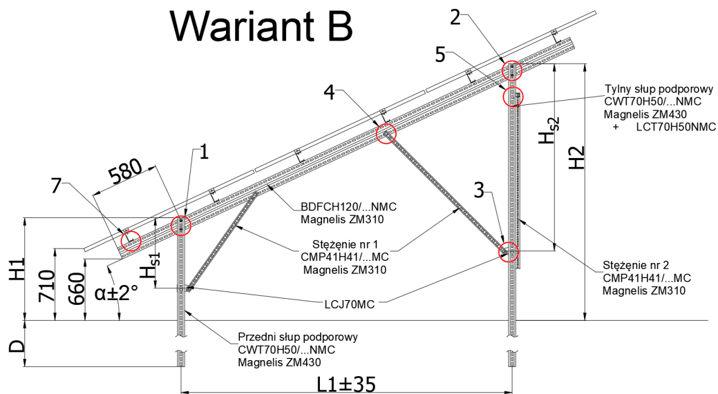
Рис. 1. Боковий вигляд конструкції
